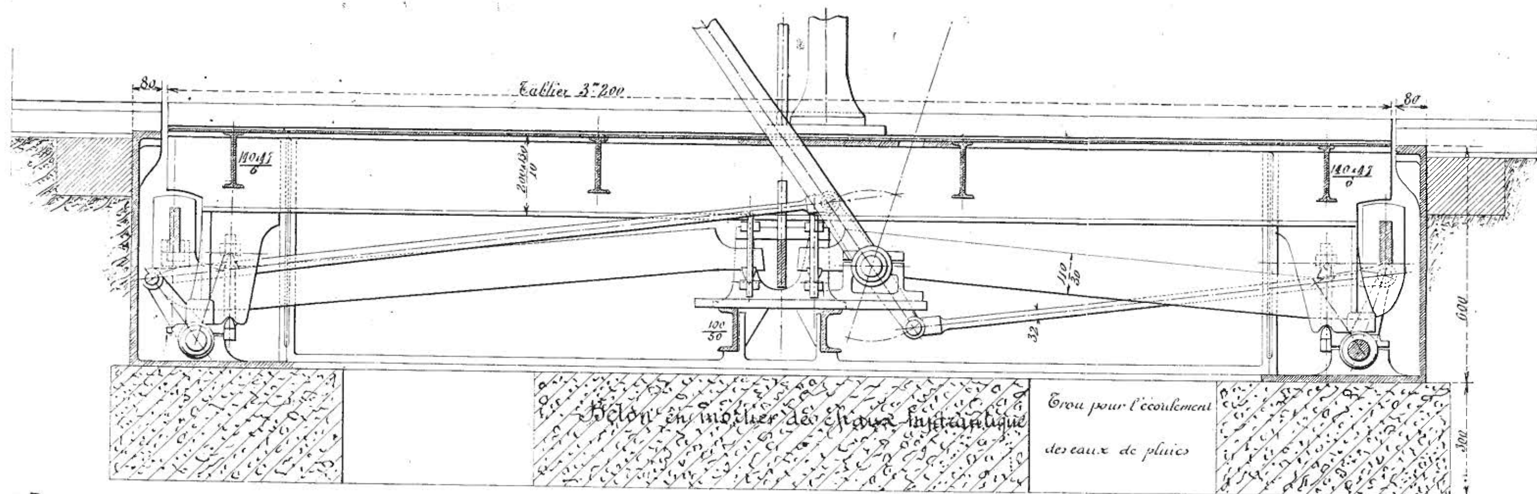
Elevation suivant AB
